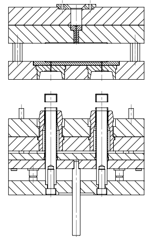
SECTION D-D
