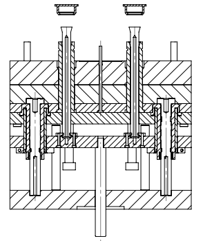
SECTION D-D
