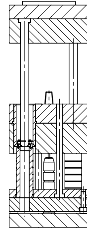
SECTION D-D
